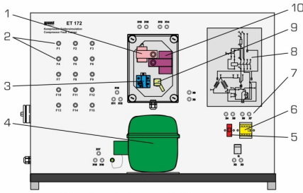
1 condensateur de service, 2 bobines-poussoirs des bornes, 3 relais de démarrage, 4 compresseur d'agent réfrigérant, 5 coupe-circuit automatique, 6 contacteur de puissance, 7 connecteurs de liaison, 8 schéma de connexion, 9 protection thermique, 10 condensateur de démarrage
